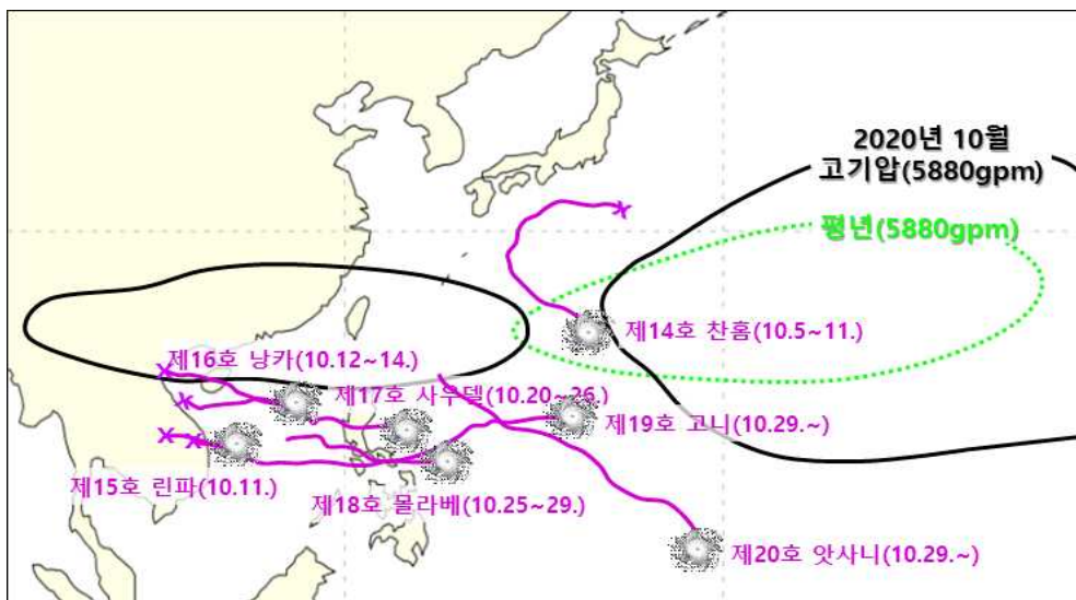
【그림 3】 2020년 10월 발생 태풍 경로와 고기압(5880gpm) 위치
