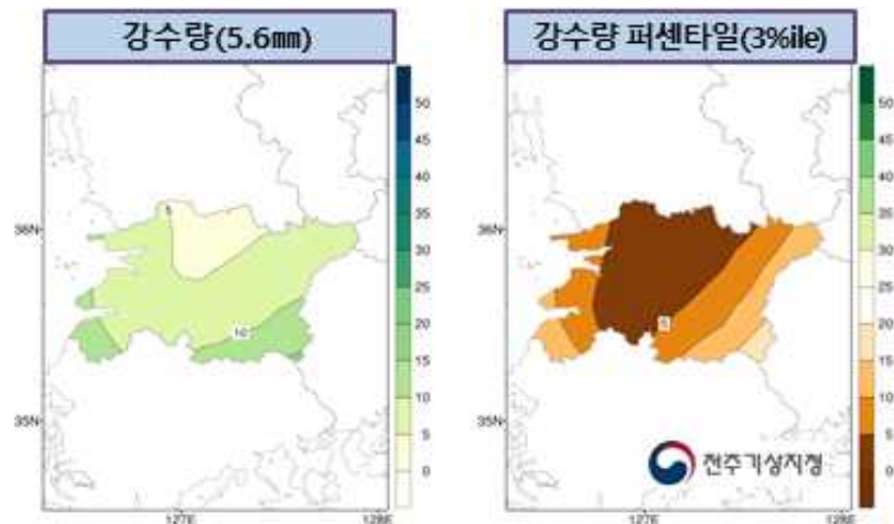
【그림 2】 2020년 10월 전북 강수량의 (왼쪽) 일변화 시계열과 (오른쪽) 분포도
