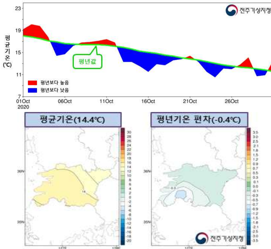
【그림 1】 2020년 10월 전북 평균기온의 (왼쪽) 일변화 시계열과 (오른쪽) 분포도
