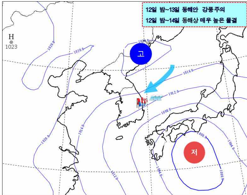
[ 4월 12일 21시 기압계 모식도 ]
